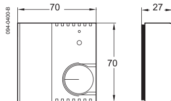
THP1+1C sonda temperatury otoczenia
