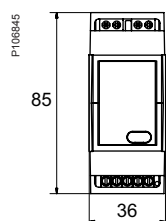
STD400RC/RL
