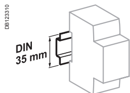
Mocowane zatraskowo na szynie DIN 35 mm
