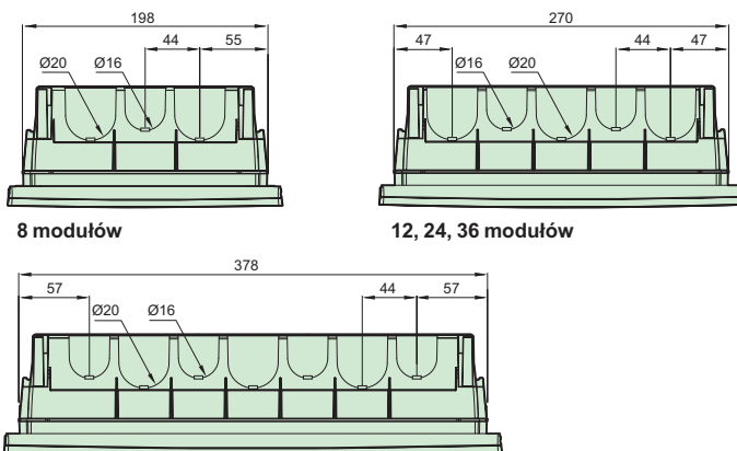
18 modułów
