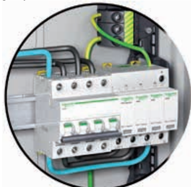
Ogranicznik przepięć iPRD 3P+N + iC60N 3P+N
