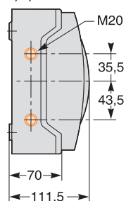
4, 6, 8 i 12 modułów
