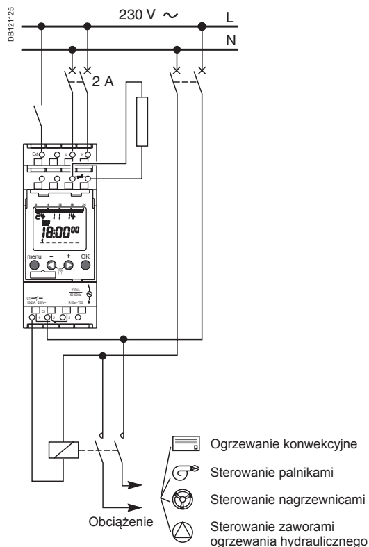
Rys. 5. THP1 +1C przykład połączenia.
