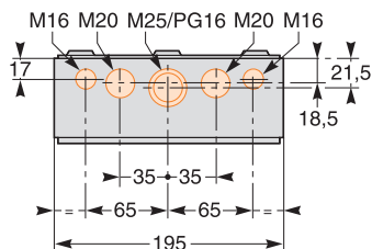
8 modułów
