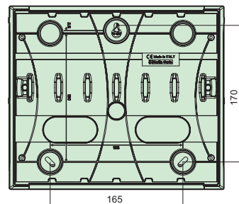
12 modułów
