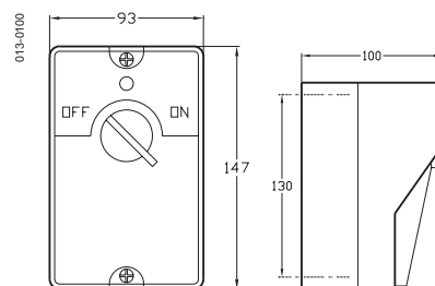
Obudowa izolacyjna
