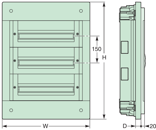
Obudowa
