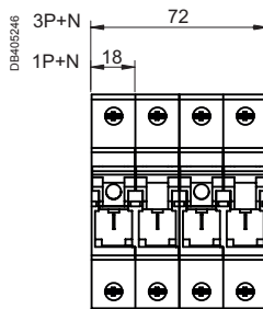
Rozłączniki bezpiecznikowe D01
