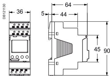
Termostat programowalny THP1+1C
