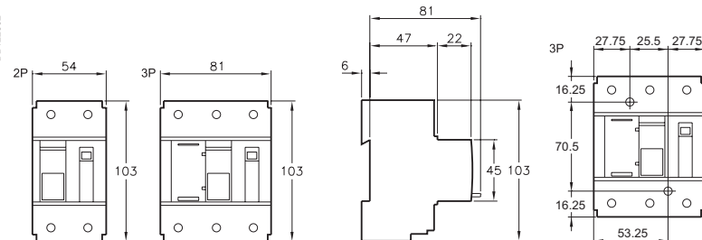
Przy montażu panelowym należy zachować odstępy
