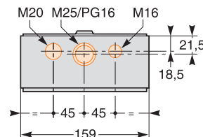
6 modułów
