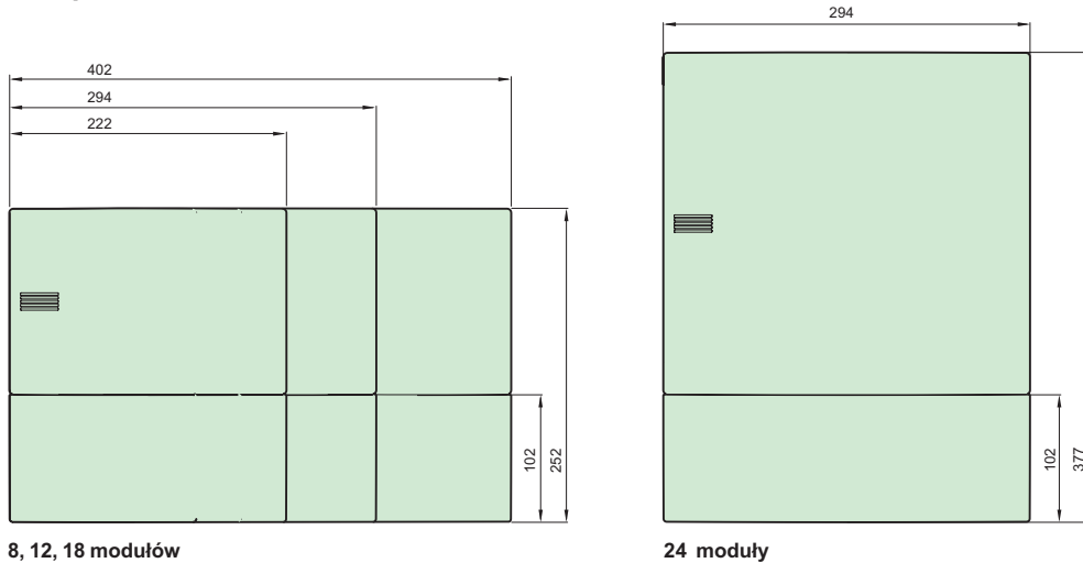
8, 12, 18 modułów
