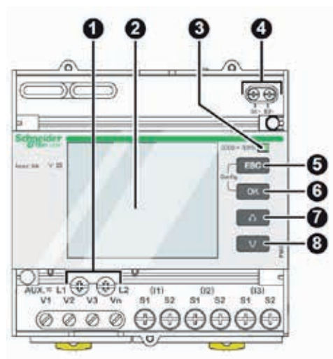
Miernik PM3255
