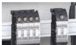
Możliwość przekształcenia listwy zaciskowej w blok rozdzielczy zasilający do 125 A, przy wykorzystaniu wspornika PRA90048.
