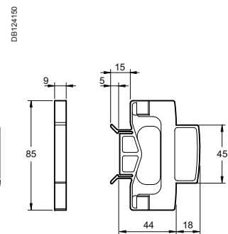
Odstępnik
