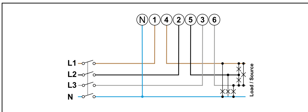
3 fazy, 4 przewody
