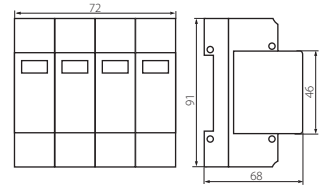
KSD-T2 275/160 3P+N
