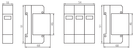
KSD-T2 275/40 1P
