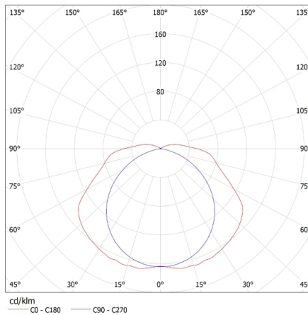
MILEDO (kat 31062) DICHT 4LED N 236/PS i T8 Miledo / LDC (Polar)
