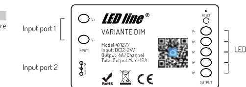
Abb.1 Controller-Ansicht
