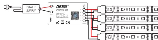
Rys.2 Schemat instalacji
