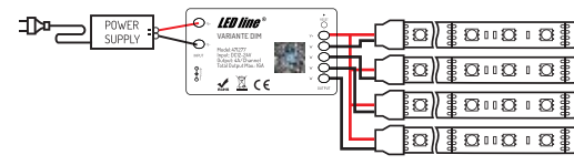
Abb. 2 Installationschema
