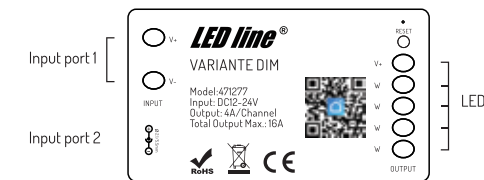
Rys.1 Widok kontrolera
