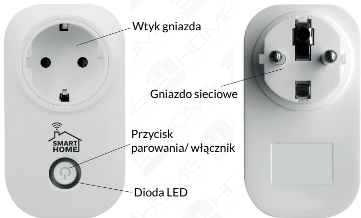
Rys. 1. Budowa i opis WS-31H1
