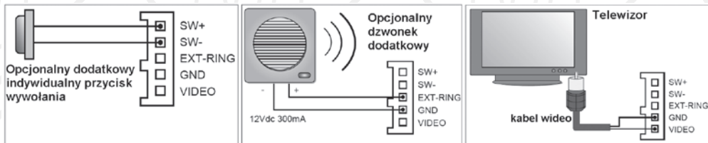
Rys.26. Opcjonalne podłączenie dodatkowych urządzeń do monitora zestawu
