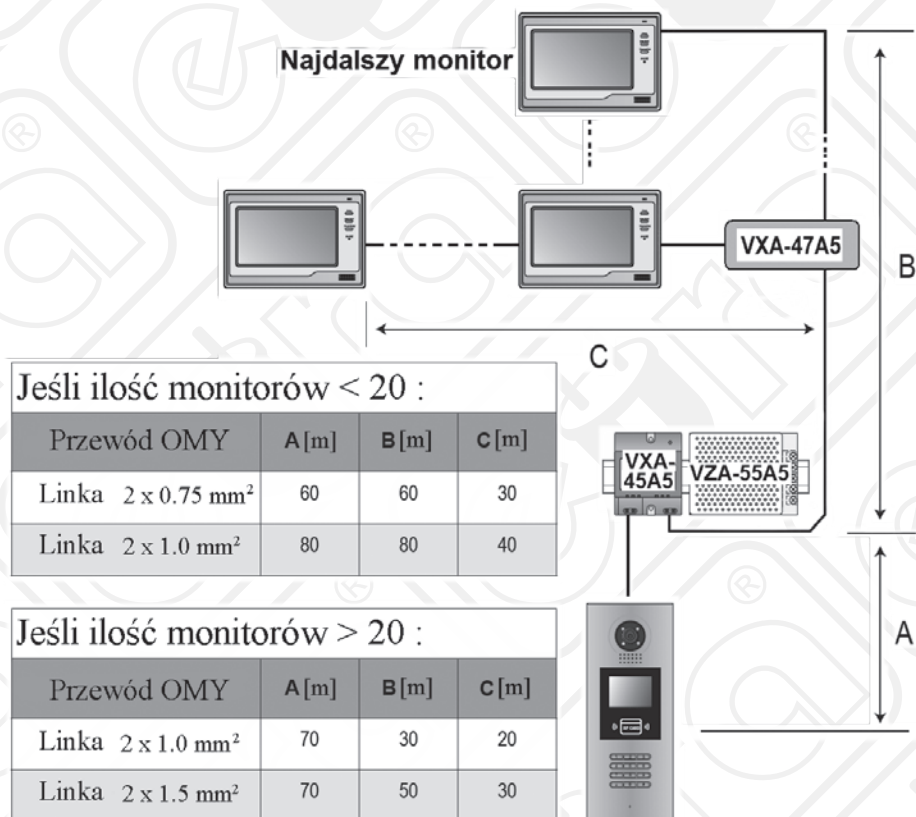
Rys.7. Dobór długości przewodów w systemie EURA-2EASY
