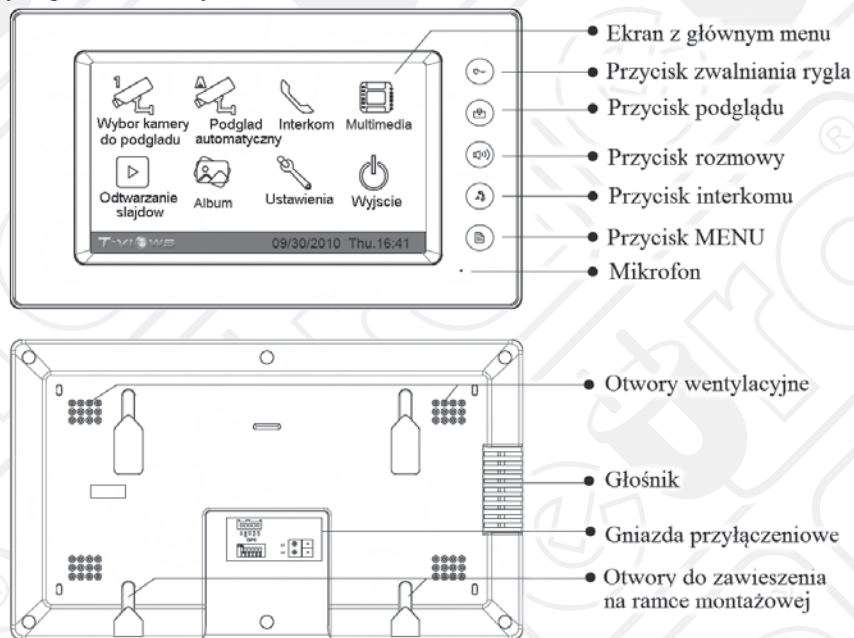
Rys.3. Widok zewnętrzny monitora VDA-09A5
