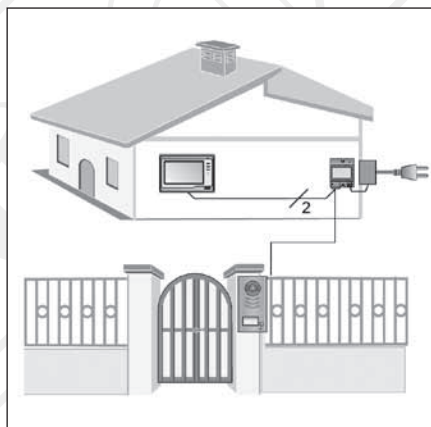
Rys.1. Konfiguracja systemu w budynku 1-lokatorskim z kasetą VDA-14A5
