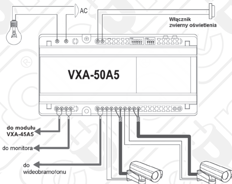
Rys.27. Opcjonalne podłączenie do wideodomofonu kamer monitorujących CCTV oraz oświetlenia zewnętrznego z wykorzystaniem modułu sterownika VXA-50A5 (element wyposażenia dodatkowego).
