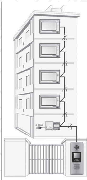
Rys.2. Konfiguracja systemu w budynku wielorodzinnym z kasetą VDA-15A5
