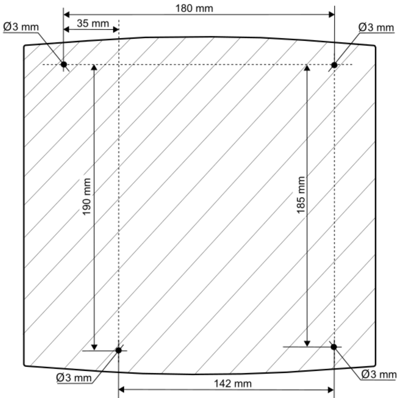
Instalacja modułu.
