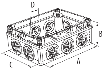
Wymiary A, B, C są wymiarami wewnętrznymi S-BOX Dimensions A, B, C – are inside dimensions of S-BOX
