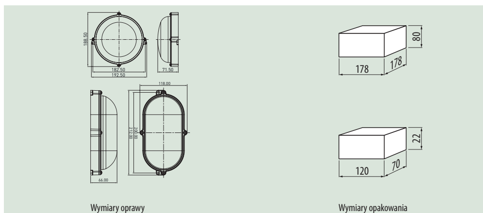
Wymiary oprawy
