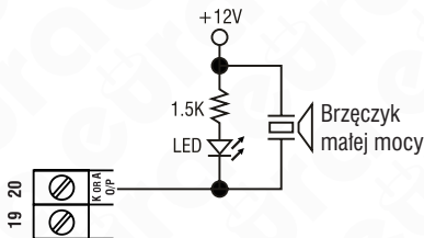
Rys. 14. Podłączenie wyjścia alarmowego prostego brzęczyka i diody LED, które dźwiękiem i światłem przez 10 sekund potwierdzą wciśnięcie dowolnego klawisza na klawiaturze
