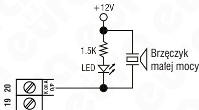
Rys. 13 Podłączenie wyjścia alarmowego zamka do prostego brzęczyka i diody LED.
