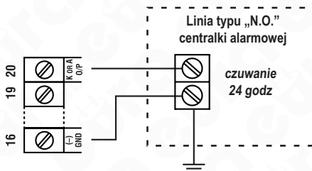
Rys. 12. Podłączenie wyjścia alarmowego zamka do zewnętrznej centralki alarmowej
