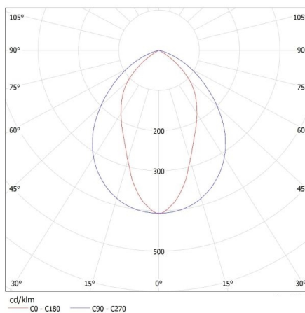
KANLUX S.A. (kat 19733) NOTUS 3 EVG 218 NT / Krzywa rozsyłu światła (biegunowo)
