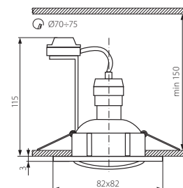
TESON AL-DTL50
