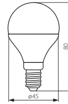
BILO 6,5W T SMD E14
