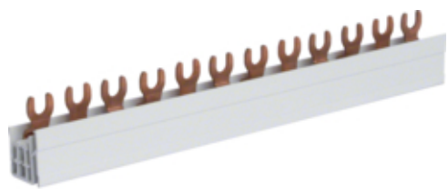
Szyna grzebieniowa widełkowa 3P, 10 mm 2 , 12M
