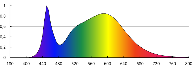
KANLUX S.A. (kat 26066) T8 LED GLASSv3 24W-NW / LDC (Polar)
